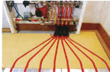
68. Zulässige Heizkreislängen
