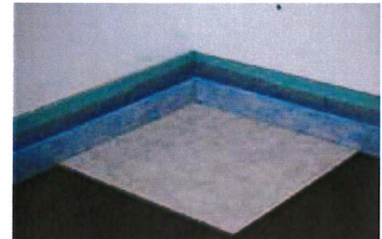
86. Bauteiltrennung
