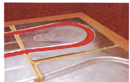
54. Richtige Lage von Rohrbögen
