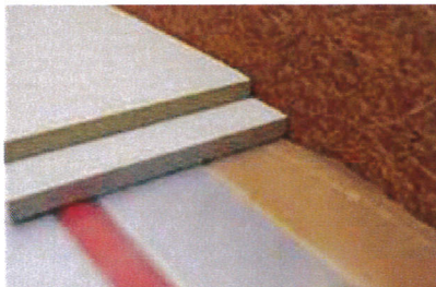
23. Geprüfte trockene Lastverteil- schichten
