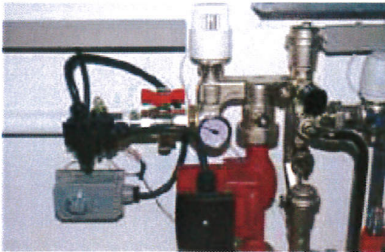
67. Belegreifheizen
