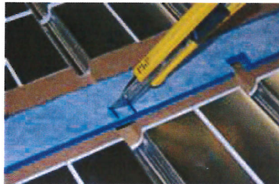
50. Bearbeiten des Dehnstreifens
